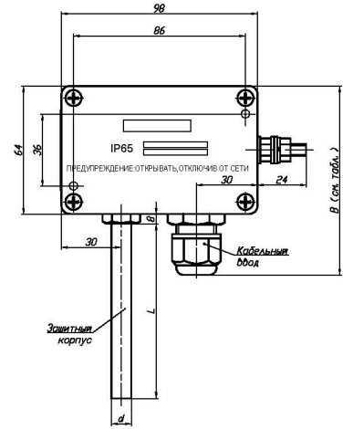
ТСп (ТС.К, ТС.П) с головкой типа «Г8/1ПРТ»: Г8/1ПРТ/Оп, Г8/1ПРТ/Ек1 (материал головки - алюминиевый сплав)
