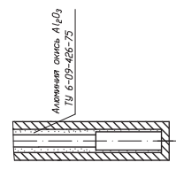
Для всех моделей ТСПУ 015. В, ТСПУ 015. 08 и ТСПУ 014, ТСПУ 015 с диапазоном нагревами до +500°С
