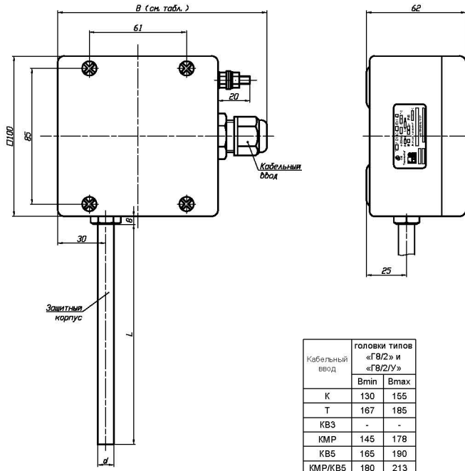
ТСп (ТС.К, ТС.П) с головкой типа «Г8/2Н»: Г8/2/Оп, Г8/2/Ех1 (материал головки - нержавеющая сталь)
