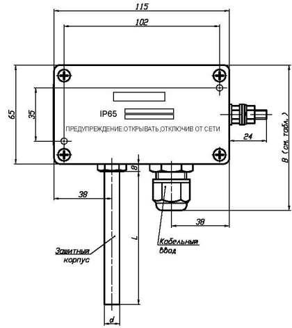
ТСп (ТС.К, ТС.П) с головкой типа «Г8/1ПРТ/У»: Г8/1ПРТ/У/Оп, Г8/1ПРТ/У/Ек1 (материал головки - алюминиевый сплав)
