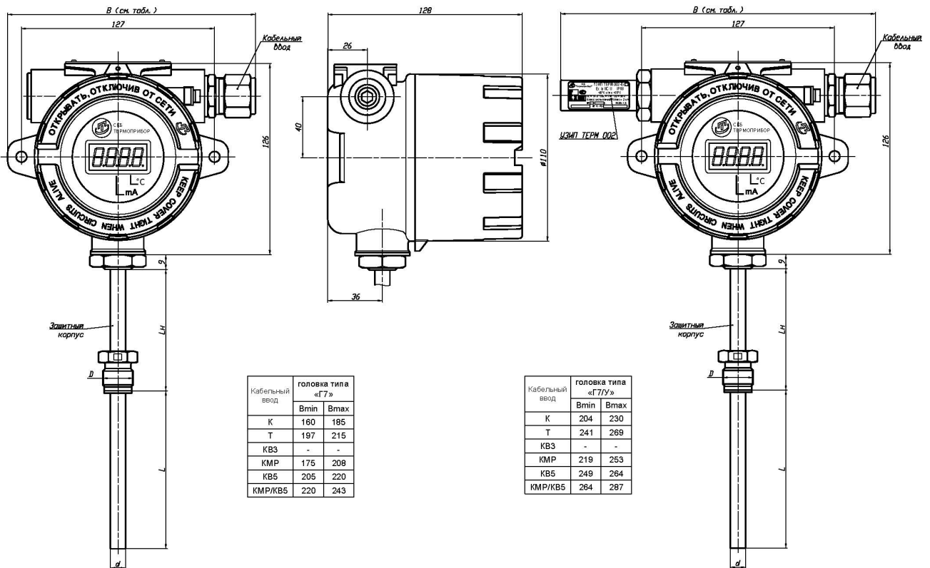
Рисунок Г.2 - Общий вид ТС (ТС.К, ТС.П) с головками типов «Г6», «Г6У» и ТС.ИНД (ТС.К.ИНД, ТС.П.ИНД) с головками типов «Г7», «Г7У»
