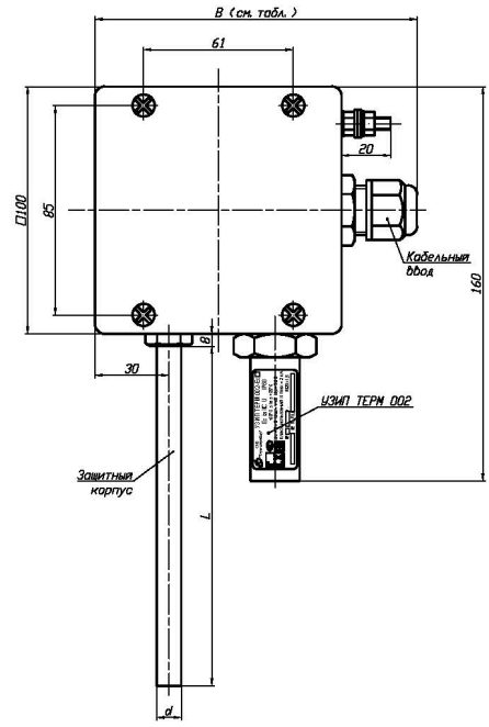
ТСп (ТС.К, ТС.П) с головкой типа «Г8/2Н»: Г8/2/Оп, Г8/2/Ех1 (материал головки - нержавеющая сталь)
