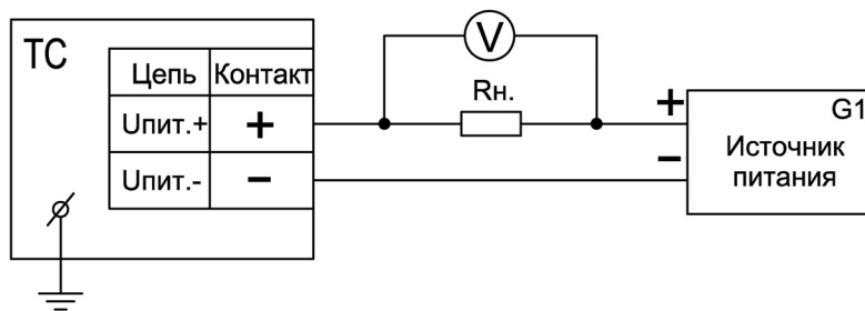
Рисунок 2.3 – Схема подключения ТС к источнику питания G1, сопротивлению нагрузки Rн. и вольтметру V
