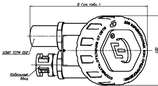
ТС с головкой типа «М(Д)»: М(Д)/Оп, М(Д)/Ех1 (материал головки - алюминиевый сплав)
