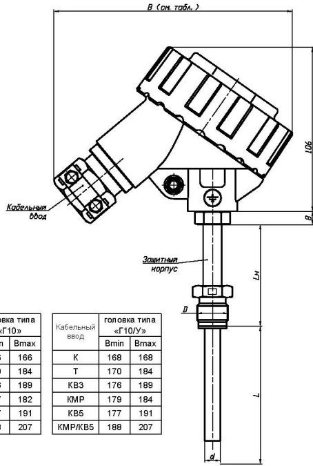
ТС с головкой типа «Г10/У»: Г10/У/Оп, Г10/У/Ехд, Г10/У/Ех1, Г10/У/Ехд1 (материал головки - алюминиевый сплав)
