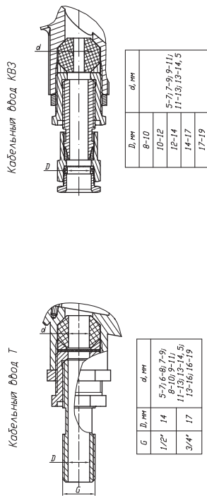
Варианты кабельного ввода с поддержанием непрерывности цепи заземления
