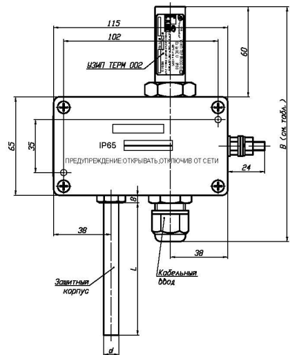
ТСп (ТС.К, ТС.П) с головкой типа «Г8/1ПРТ/У»: Г8/1ПРТ/У/Оп, Г8/1ПРТ/У/Ек1 (материал головки - алюминиевый сплав)
