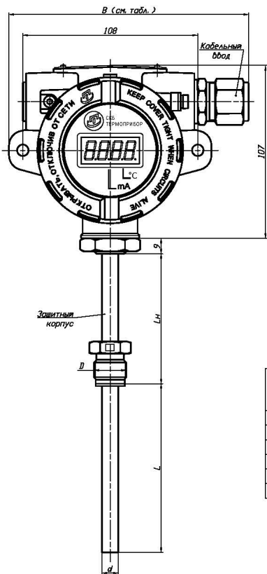
Рисунок Г.3 - Общий вид ТС (ТС.К, ТС.П) с головками типов «Г6/1», «Г6/1/У» и ТС с головками типов «Г7/1», «Г7/1/У»
