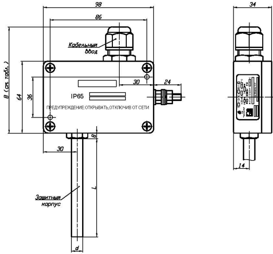
ТСп (ТС.К, ТС.П) с головкой типа «Г8/1»: Г8/1/Оп, Г8/1/Ек1 (материал головки - алюминиевый сплав)
