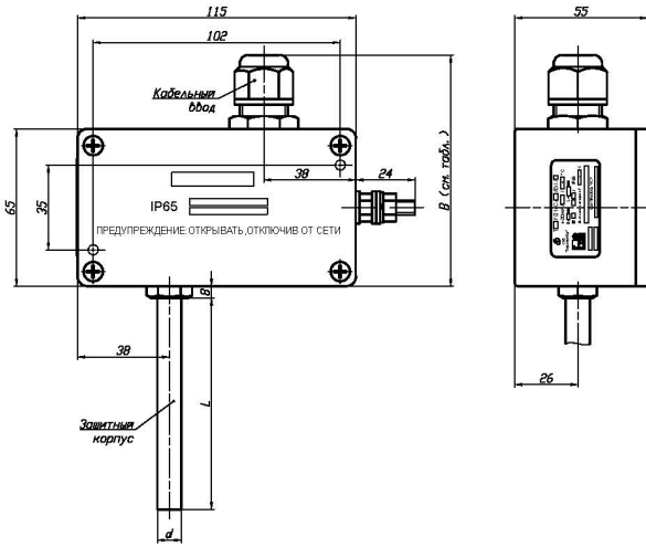
ТСп (ТС.К, ТС.П) с головкой типа «Г8/1У»: Г8/1У/Оп, Г8/1У/Ек1 (материал головки - алюминиевый сплав)
