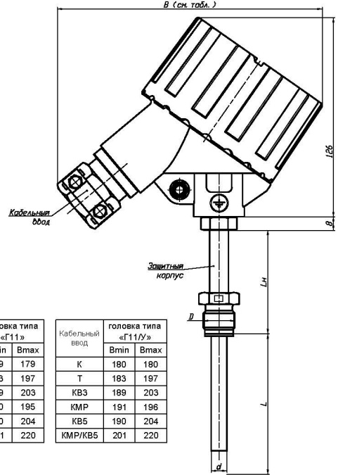
ТС.ИНД с головкой типа «Г11/У»: Г11/У/Оп, Г11/У/Ехд, Г11/У/Ех1, Г11/У/Ехд1 (материал головки - алюминиевый сплав)
