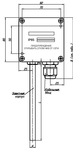
ТСп (ТС.К, ТС.П) с головкой типа «Г9ПРТ»: Г9ПРТ/Оп, Г9ПРТ/Ех1 (материал головки - поликарбонат)
