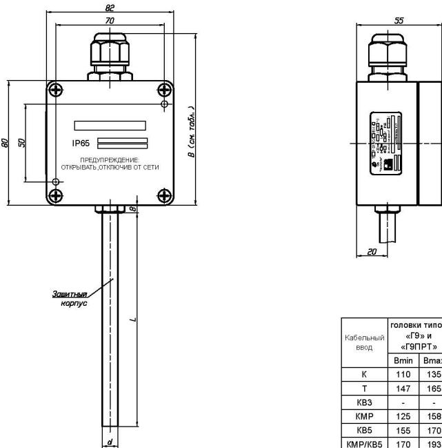
ТСп (ТС.К, ТС.П) с головкой типа «Г9»: Г9/Оп, Г9/Ех1 (материал головки - поликарбонат)
