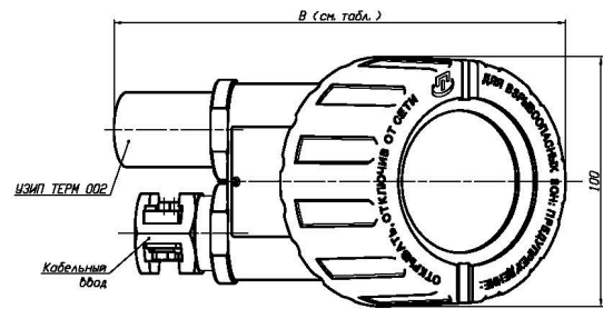
ТС с головкой типа «ПА»: ПА/Оп, ПА/Ех1 (материал головки - стеклонаполненный полиамид)
